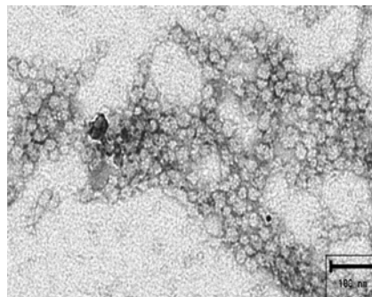
Fig. 1. Microfotografía que muestra la formación de estructuras vesiculares, después de extraer los componentes de membrana de L. interrogans serovar Canicola. Se observan abundantes partículas esféricas o vesículas de membrana externa, de tamaño homogéneo, entre 15 y 50 nm (nanoproteoliposomas). Magnificación de 60 K. Microscopio JEM1010Jeol.
