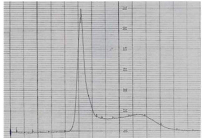
Fig. 2. Perfil cromatográfico del PLBCG mediante cromatografía de exclusión molecular. Columna XK16/40, empaquetada con Sephacryl S-1000. Se aplicó 1 mL (2 mg de proteínas) de la muestra, lo que representa aproximadamente el 1,25% del volumen total de la columna. La elución se realizó a 0,4 mL/min y se registró con un rango máximo de absorbancia de 0,2.
